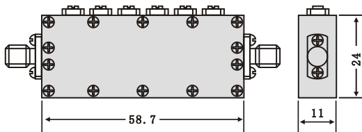
外形尺寸 Dimensions
