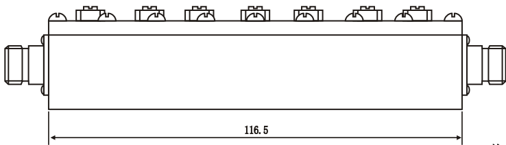
外形尺寸 Dimensions
