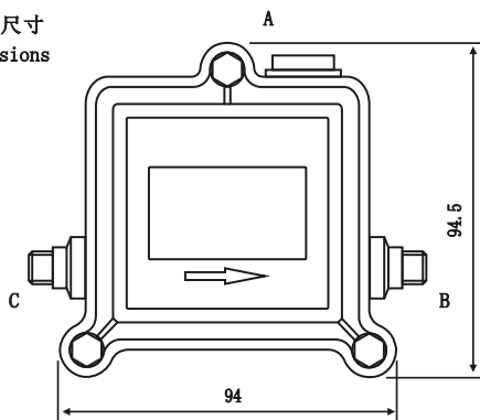
外形尺寸
