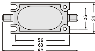
外形尺寸 Dimensions
