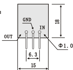
外形尺寸 Dimensions
