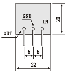
外形尺寸 Dimensions
