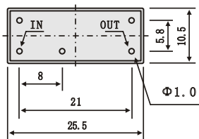
外形尺寸 Dimensions
