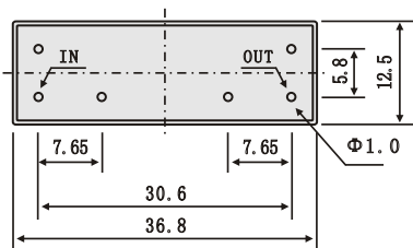
外形尺寸 Dimensions
