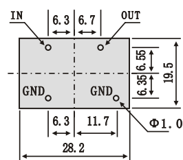
外形尺寸 Dimensions
